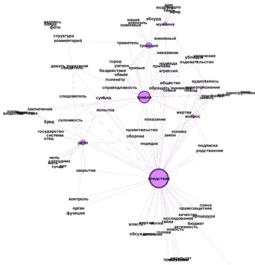
Рис. 1. Сеть понятий.
